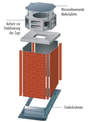
Schematischer Aufbau einer Schornsteinkopfverkleidung mit zugstabilisierendem Aufsatz.
