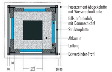
Querschnitt einer Schornsteinkopfverkleidung
