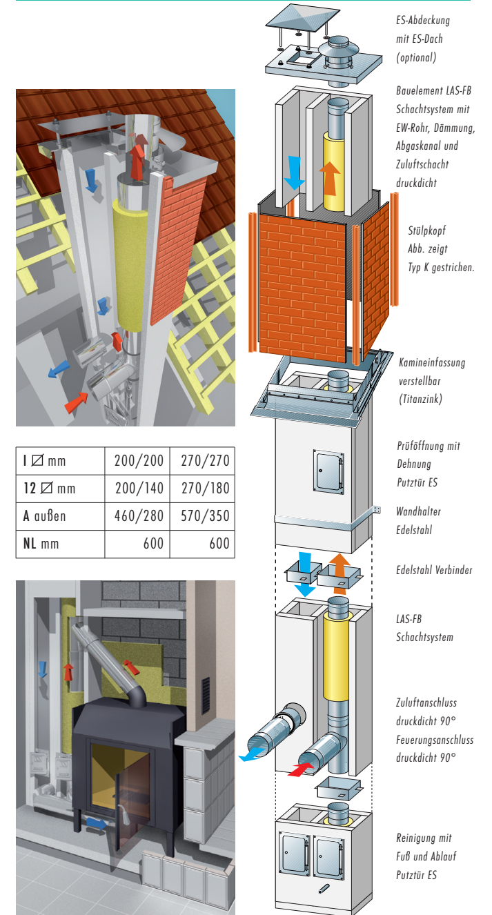
Beispielaufbau zweizügig: Abgasführung mit separater Zuluft
