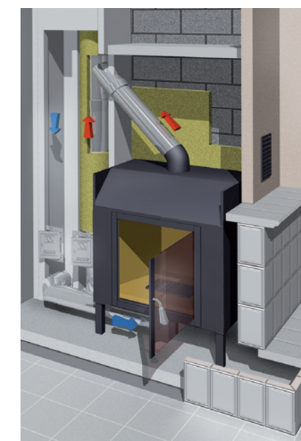
Beispielanwendung für einen Kachelofen
