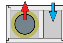
Abgas- und separater Zuluftschacht. Für raumluftunabhängige Festbrennstofföfen.
