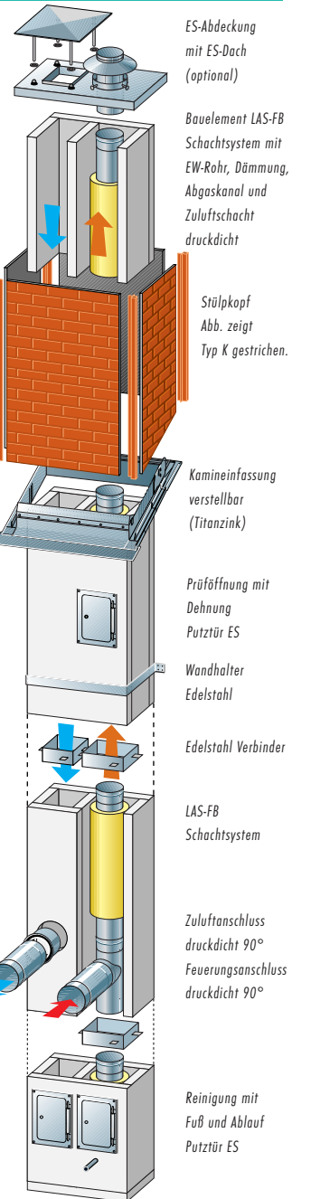
Beispielaufbau zweizügig: Abgasführung mit separater Zuluft
