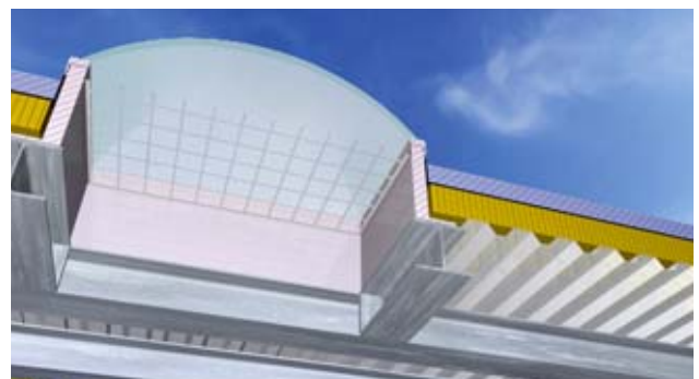
2 Dachöffnung (Lichtkuppel) mit fest eingebautem Schutzgitter als permanenter Schutz
