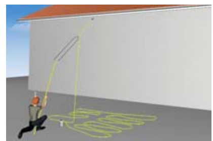
3 Seilwurfsystem zur Installation des Anseilschutzes bei kurz dauernden Arbeiten (siehe Regel 8)
