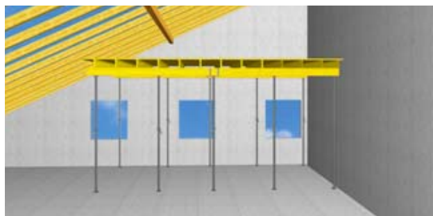
2 Fanggerüst im Aufbau. Dieses muss noch verlängert werden, bis der ganze Absturzbereich geschützt ist.
